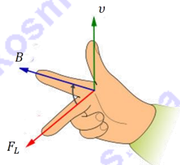
Σχ. 1 Κανόνας δεξιού χεριού
